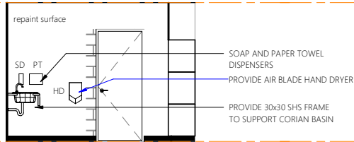
Elevation 5E
