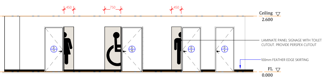
Elevation 2E 1:50
