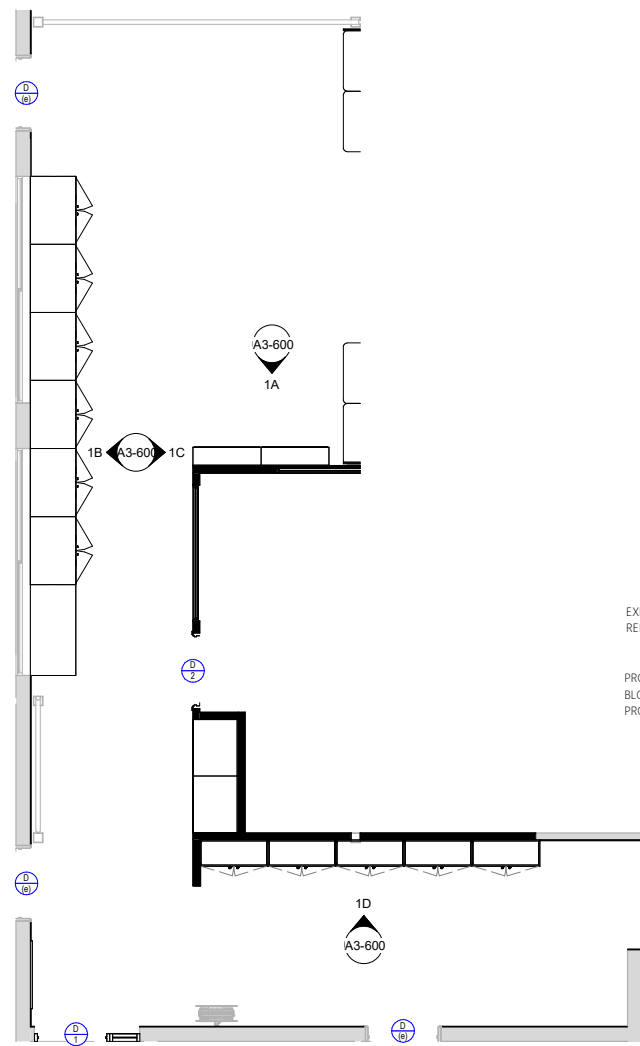
Internal Plan 1 1 : 50
