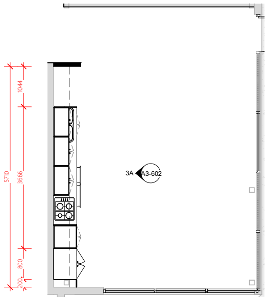
Internal Plan 3 1 : 50
