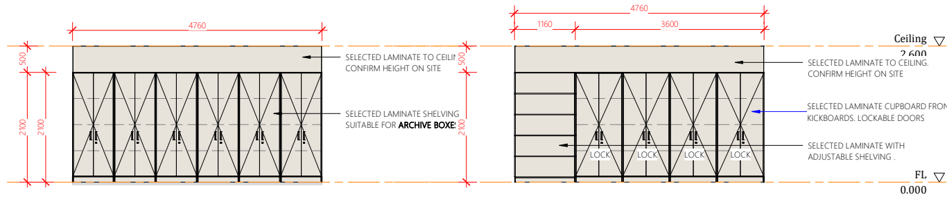
Elevation 2A 1:50
