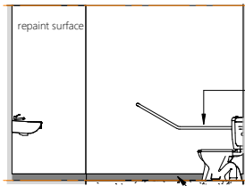
Elevation 5B
